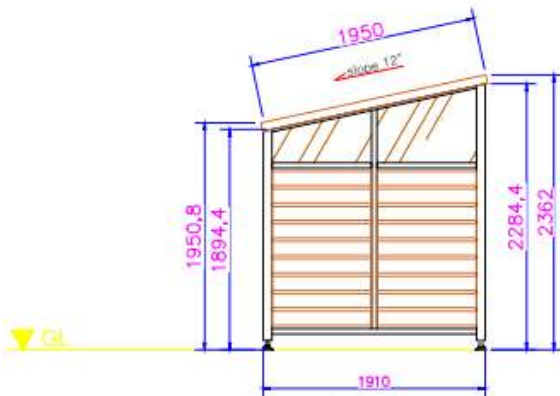
좌측면도
