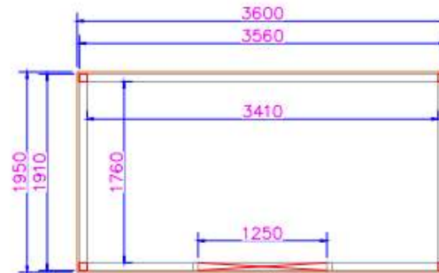
평면도
