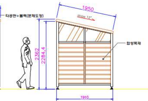
우측면도
