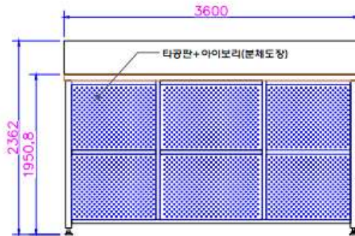
후면도
