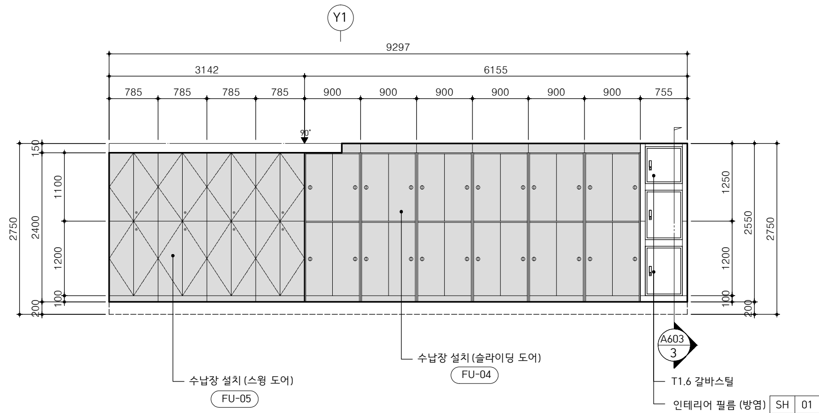
2 실습실(405호) 내부전개도-2 축 척 : 1 / 60
