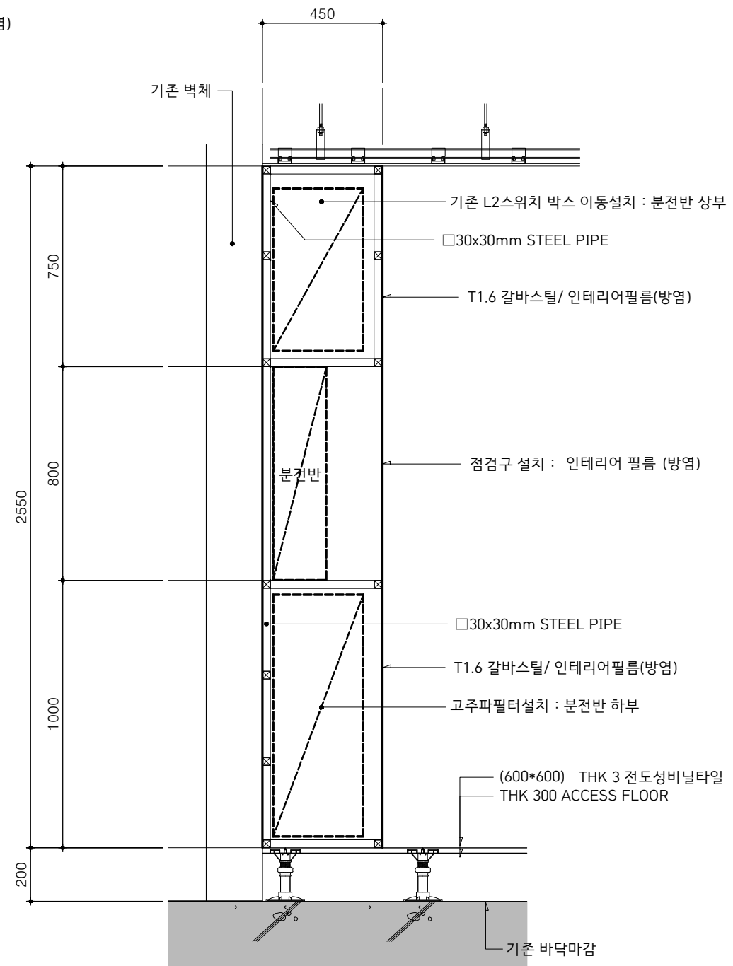
단면 상세도
