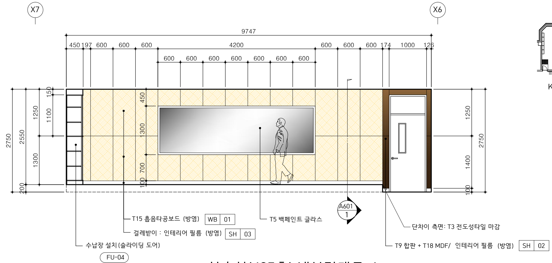
1 실습실(405호) 내부전개도-1 축척 : 1 / 60
