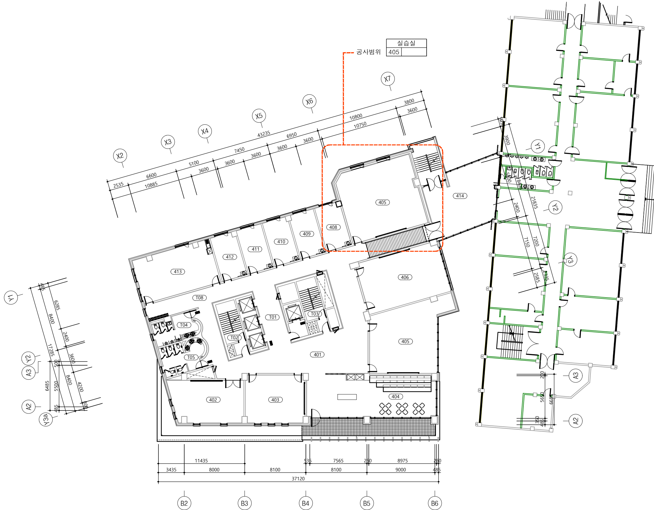
지 상 4 층 전 체 평 면 도 축 척 : 1 / 300
