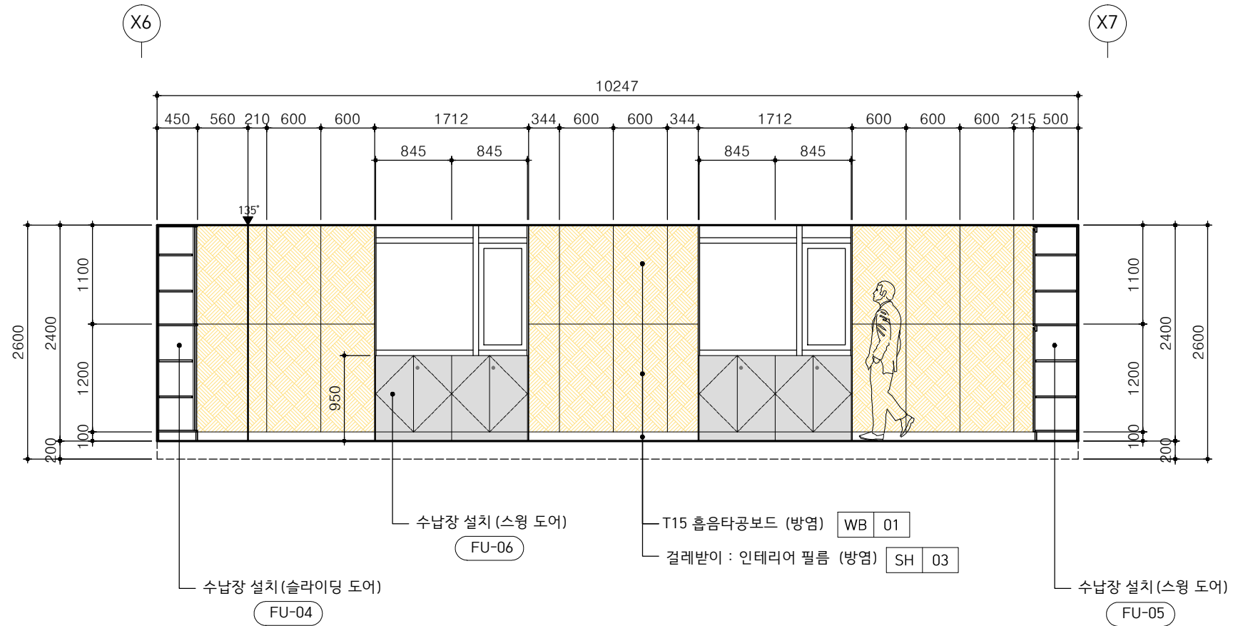
1 실습실(405호) 내부전개도-1 축 척 : 1 / 60
