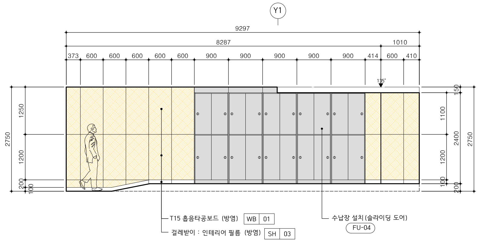
2 실습실(405호) 내부전개도-2 축척 : 1 / 60
