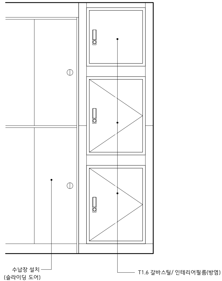
입면 상세도
