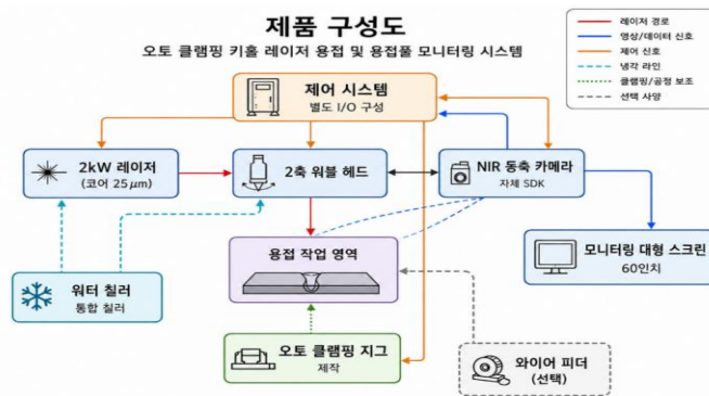
[참조 3] 제품 구성도
