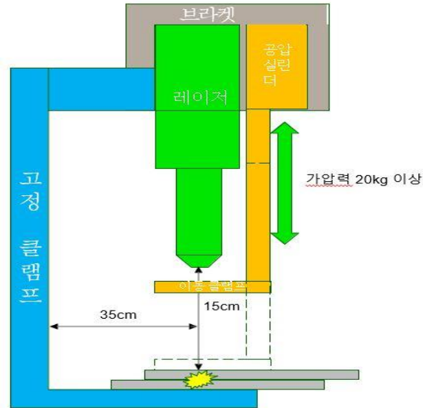
[참조 2] 오토클램핑 지그 헤드예시
