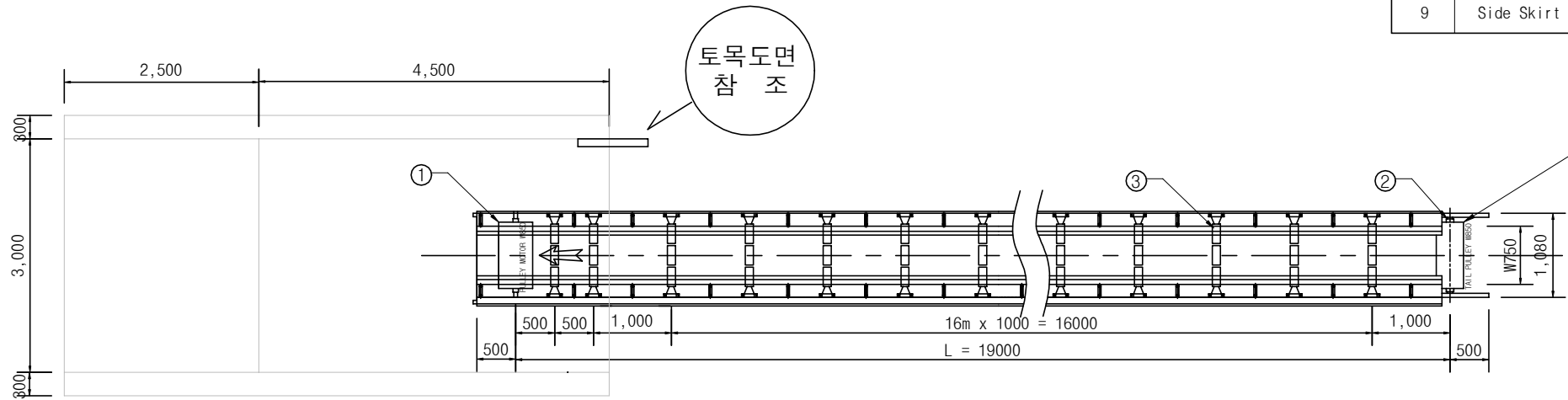
협잡물 이송컨베이어(수평형)평면도
