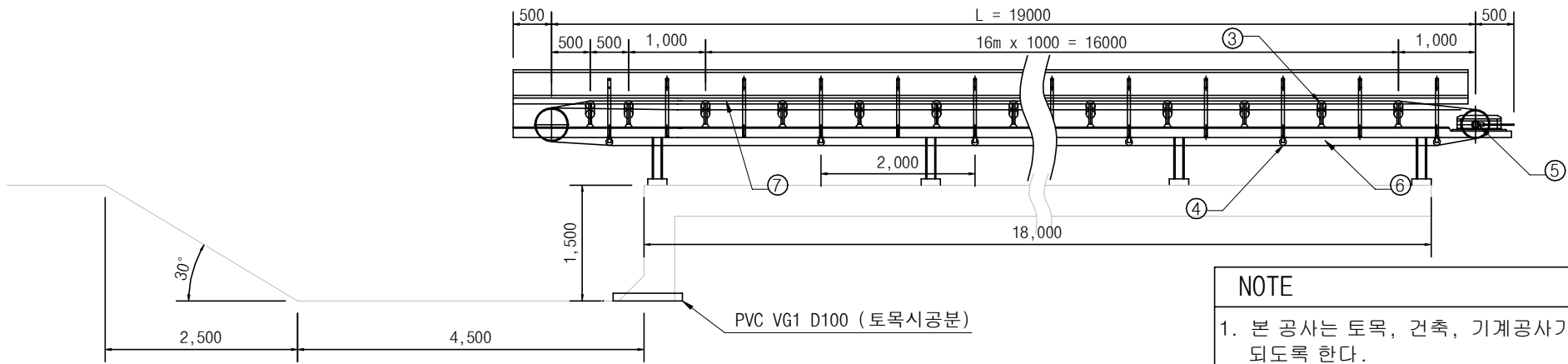
협잡물 이송컨베이어(수평형)측면도
