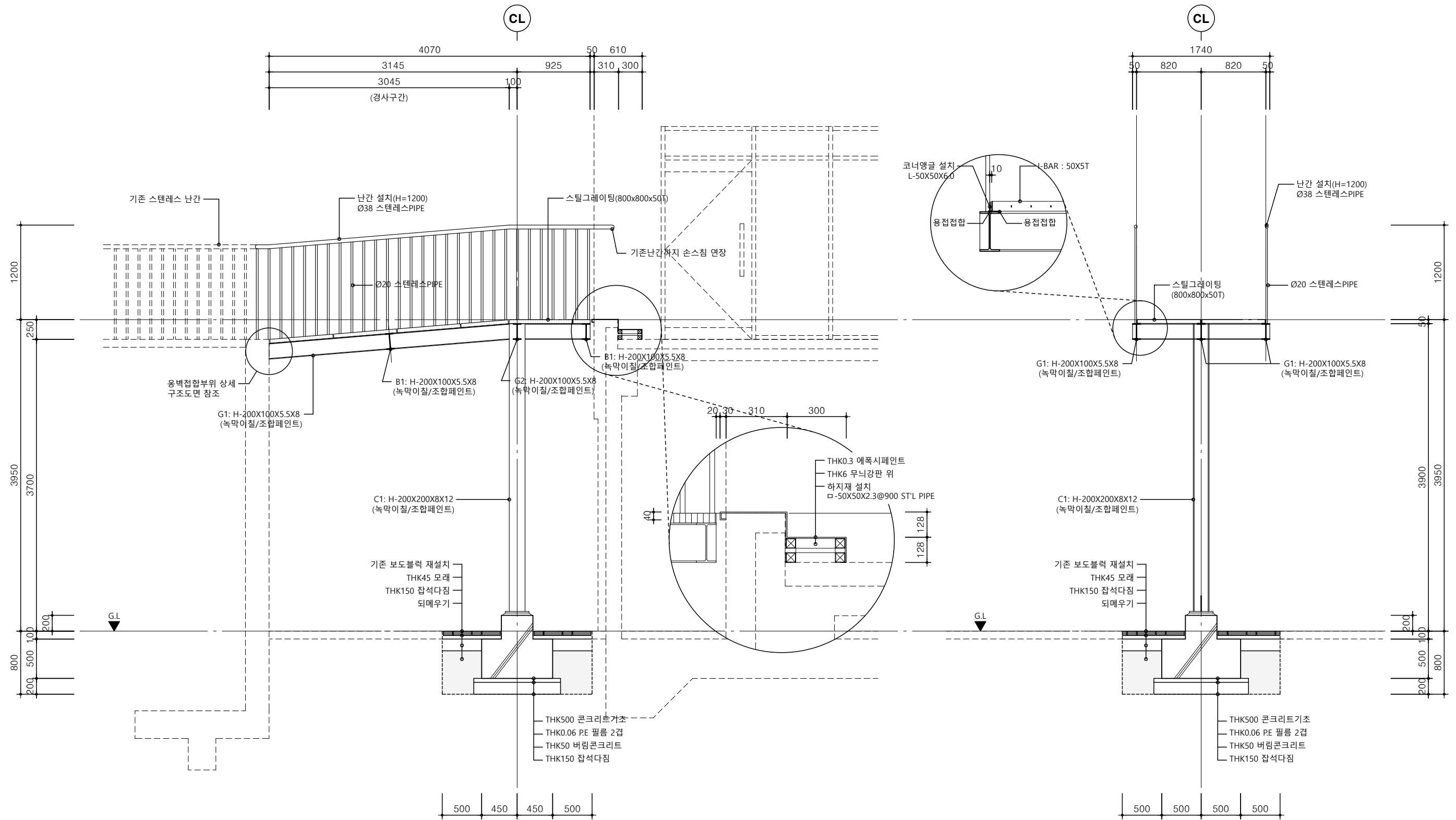
1 단면도 -1 축척 : 1/ 25 (A1) 1/ 50 (A3)
