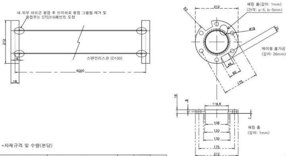
압상파이프 가공플랜지 제작도 (D100)
