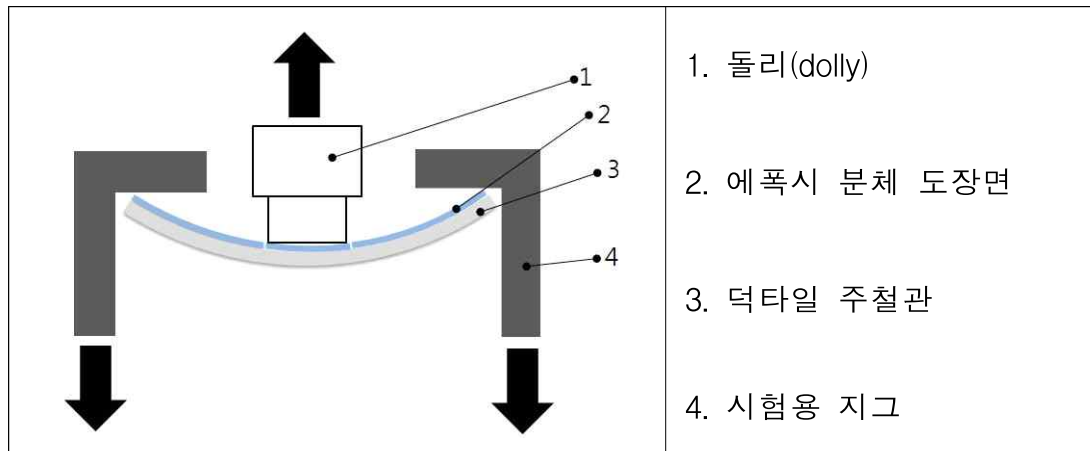
[그림5] 시험 개략도
