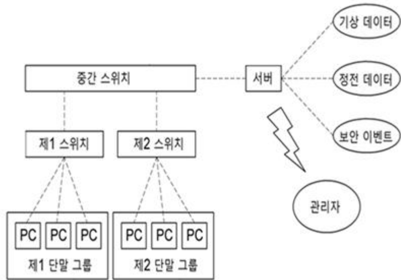
<단일 서버 기반의 이중 네트워크 장애 관리 시스템 구성도>
