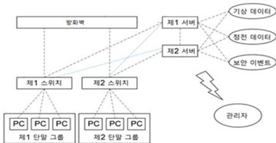
<이중 네트워크 장애 관리 시스템 구성도>
