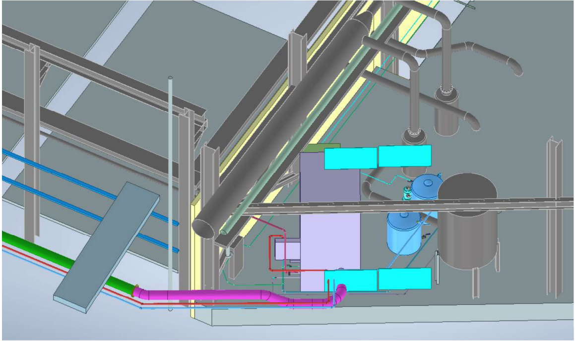
[붙임3] 준비동 설비 측면도
