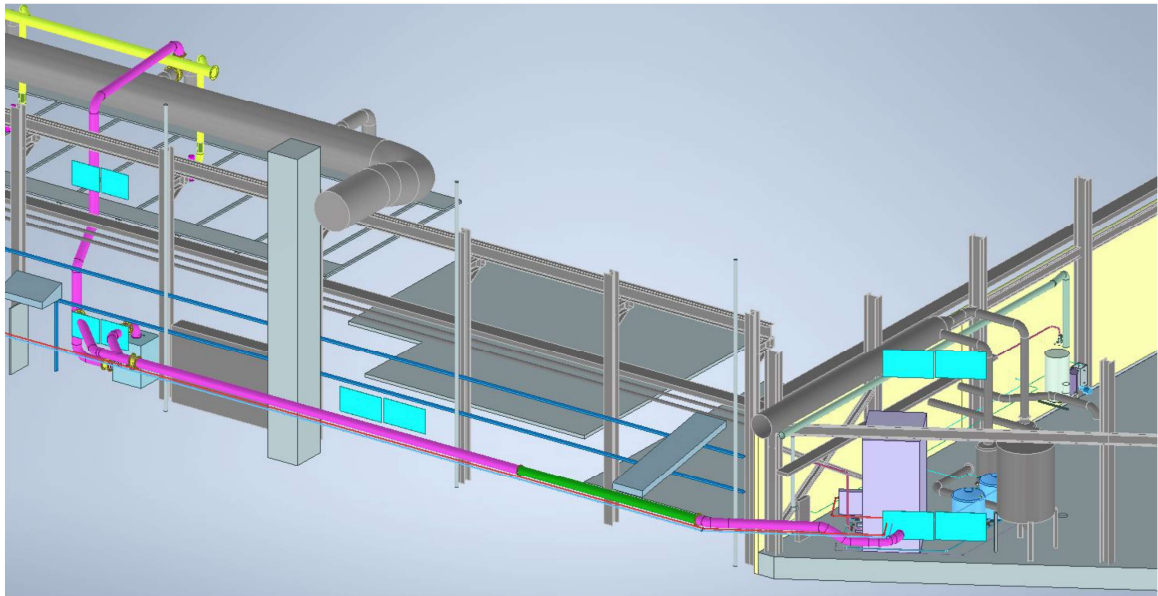
[붙임1] 공정동·준비동 설비 연동 배치도(종합)
