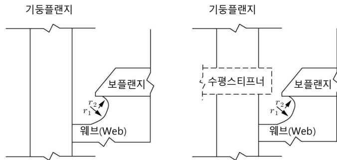
그림 3.3-2 스캘럽의 개선가공
