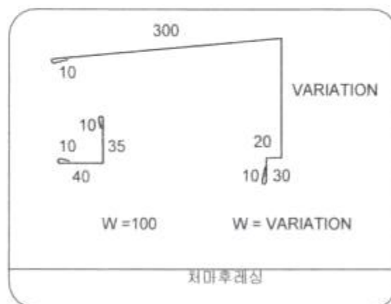
상세도 "A"
