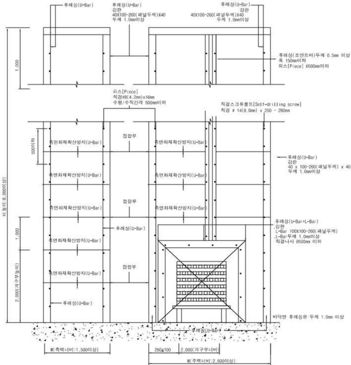
[ 주벽 및 측벽 입면도 ]
