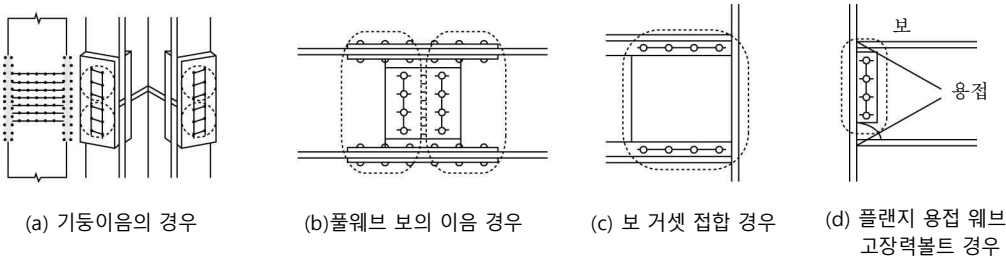
그림 3.3-1 가볼트 조임에서의 볼트 1군의 개념
