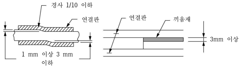
그림 3.8-2 모재의 단차
