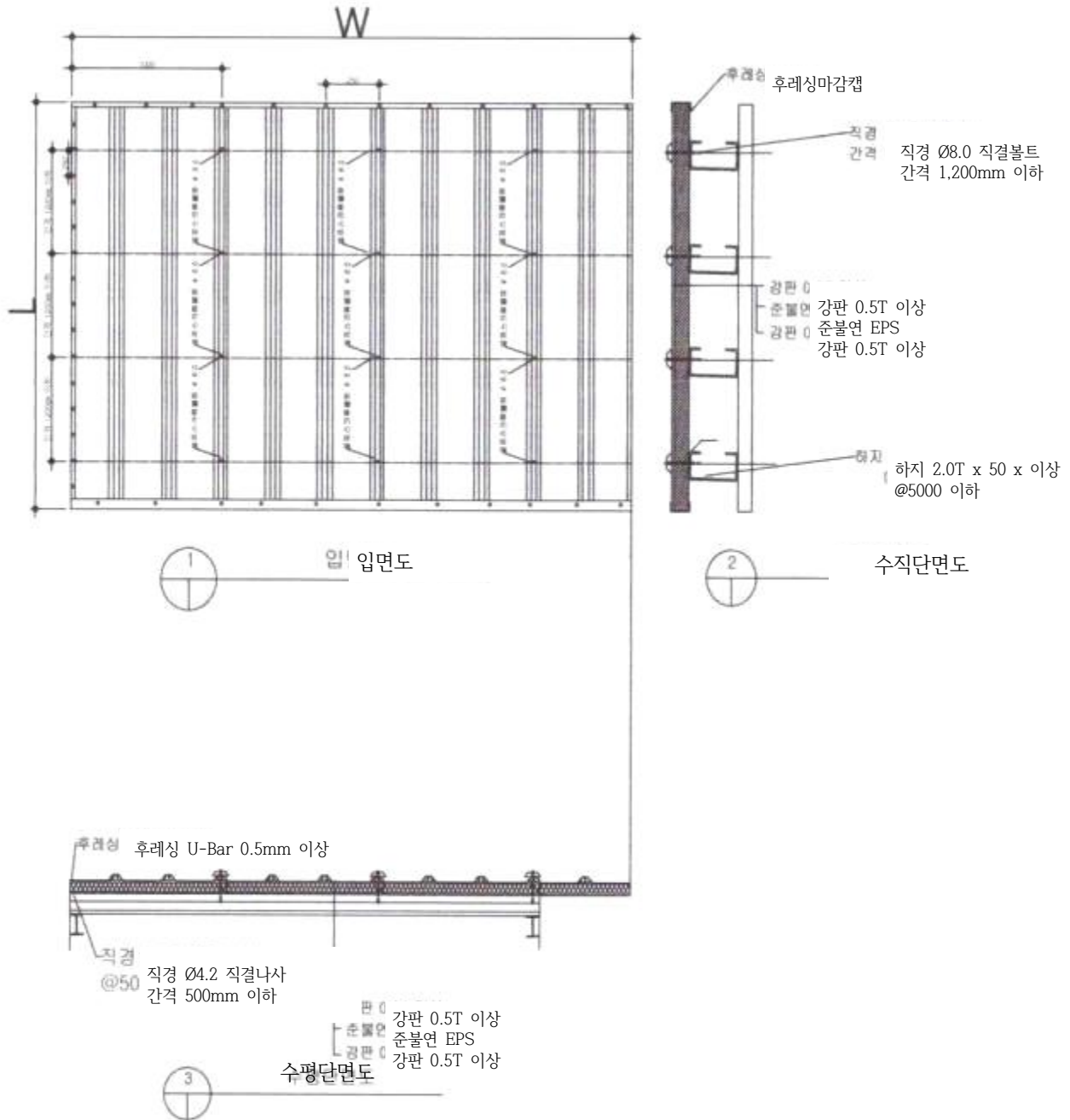
지붕판 구조 설명도
