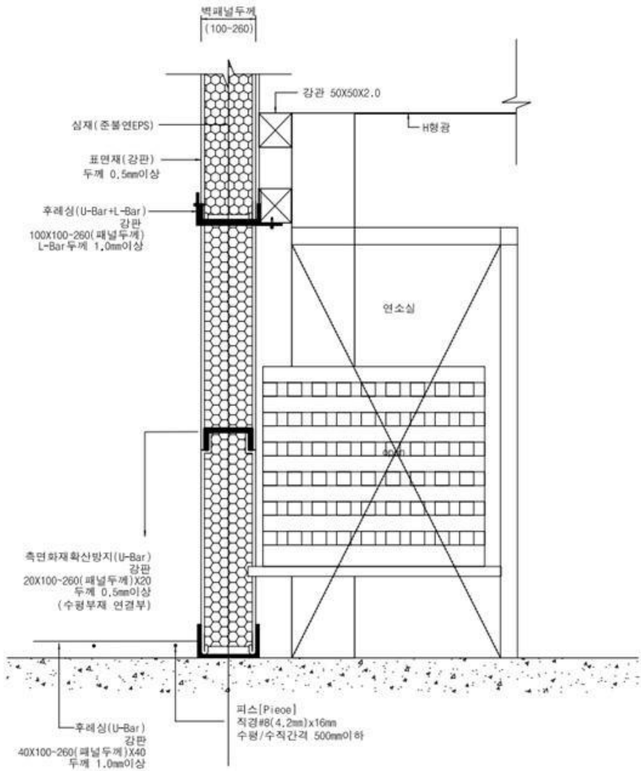
[ 개구부 주변 종방향 단면도 ]
