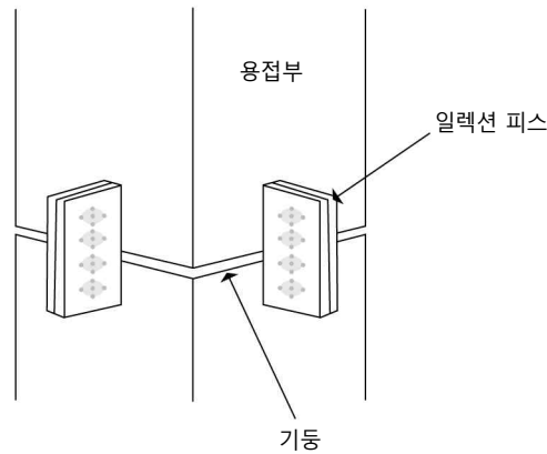
그림 3.3-2 일렉션피스의 가동
