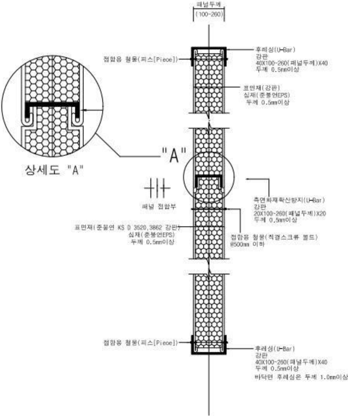
[ 구성재료 설명도 2 (수평연결부) ]
