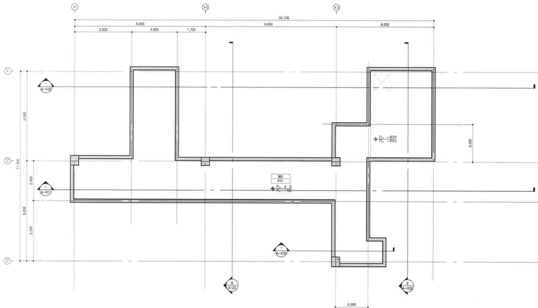
1 PIT층 평면도 축척: 1/100
